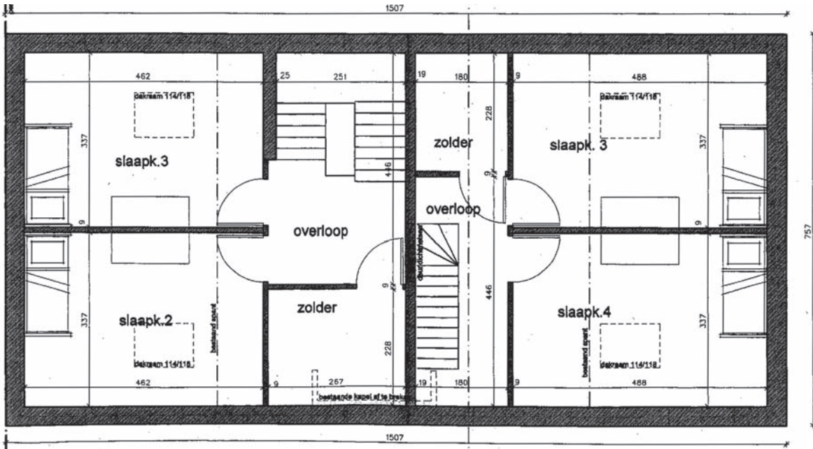
Grondplan eerste verdieping
