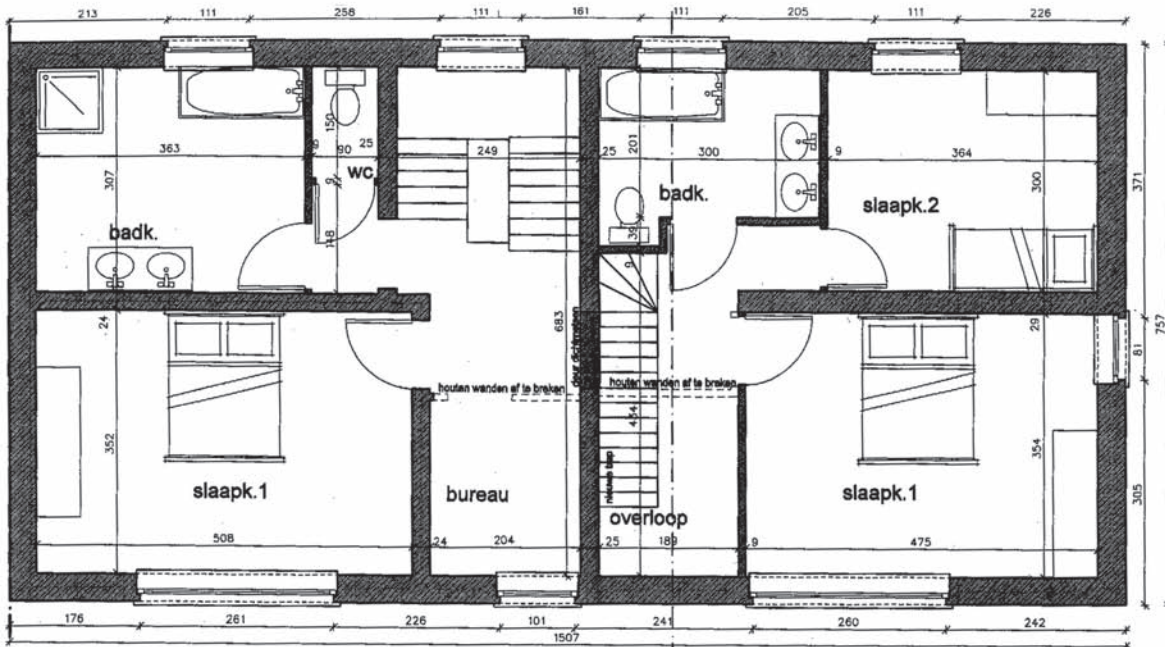
Grondplan tweede verdieping
