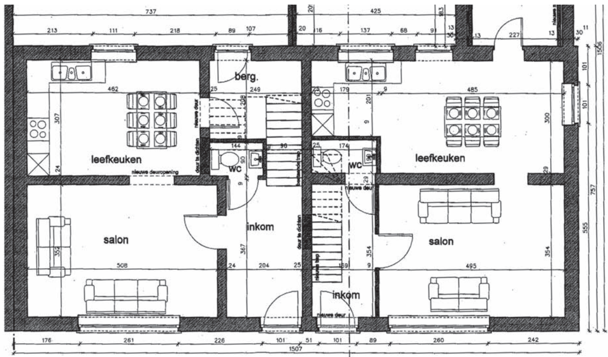
Grondplan gelijkvloers
